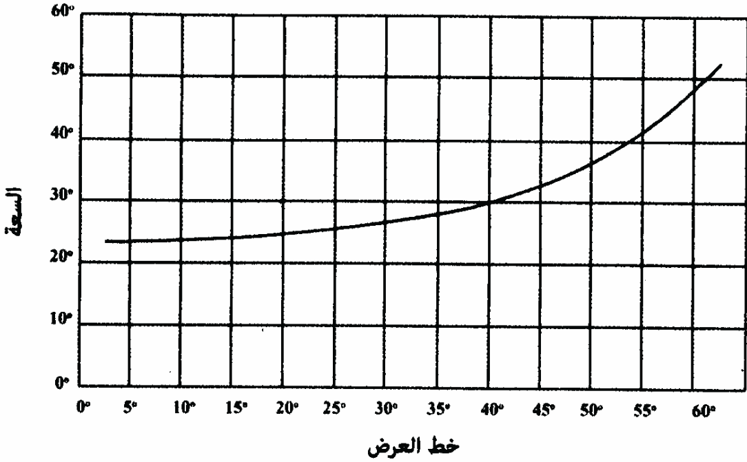
الشكل (78): تختلف سعة الشمس العظمى باختلاف خط العرض.
